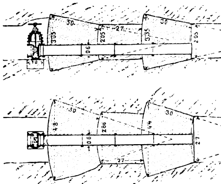
Č. 1806. Hráz v hornictví: nárys a půdorys.
